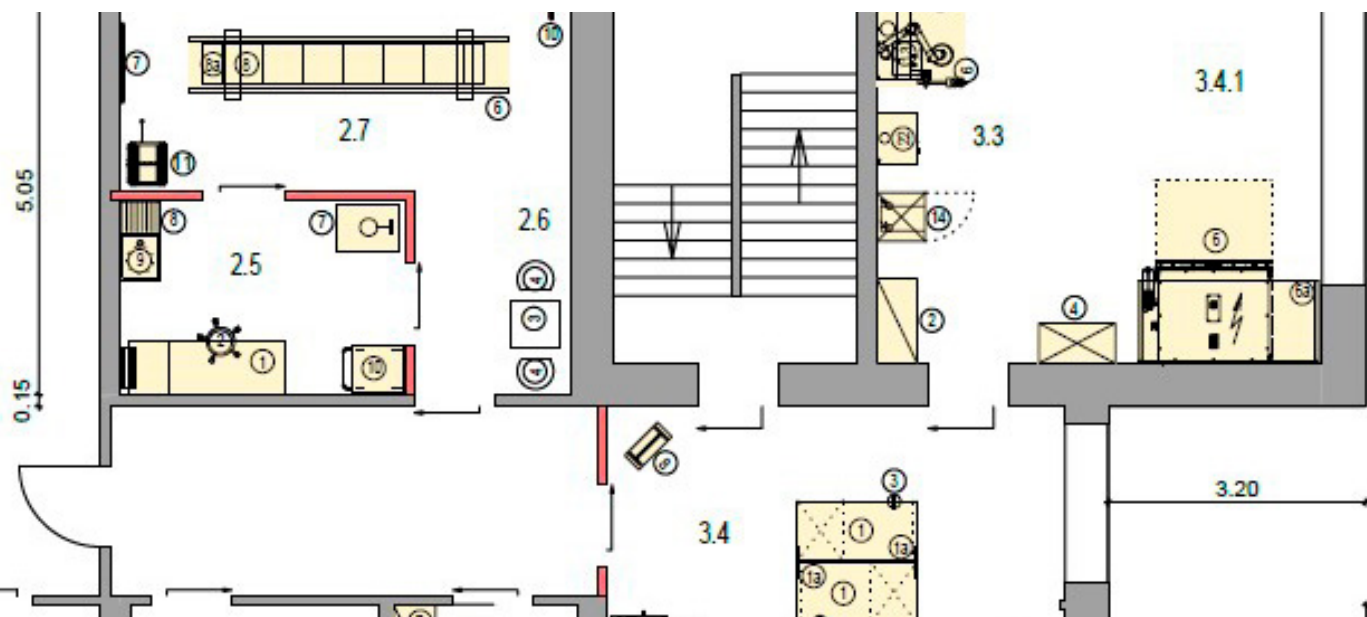
Ausschnitt des Werkstattaufbauplans
